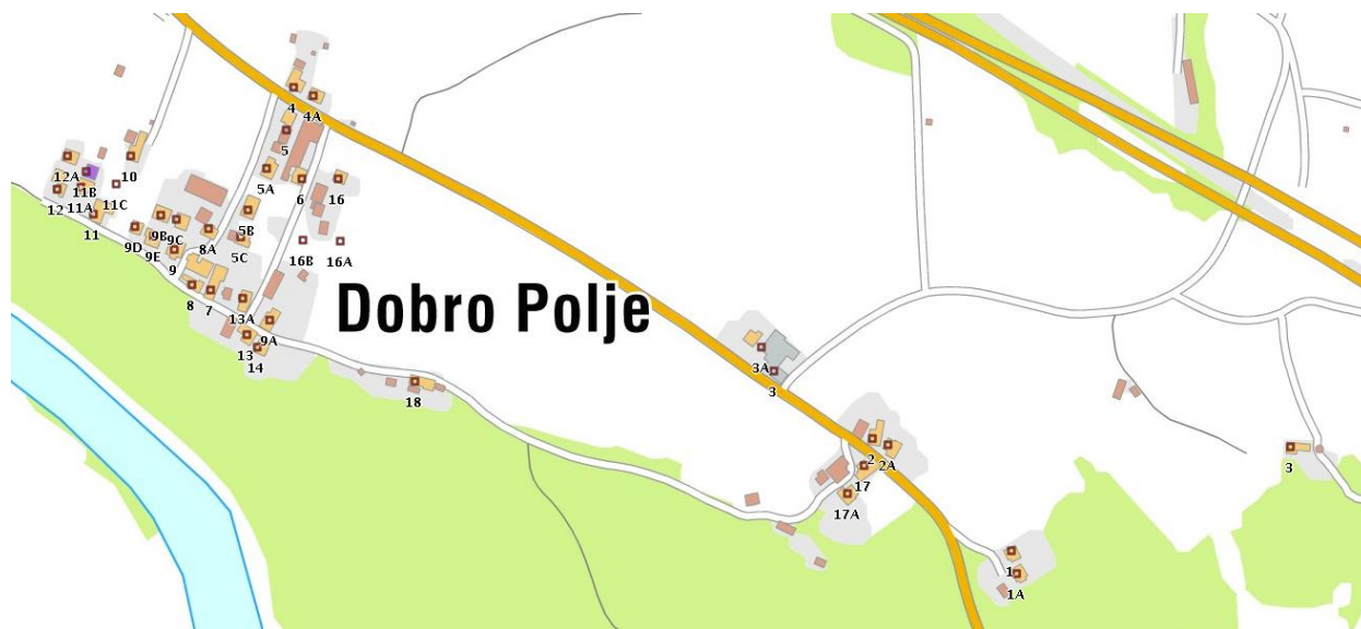
Dobro Polje – topografska karta, 2016 Vir: geopedija.si
